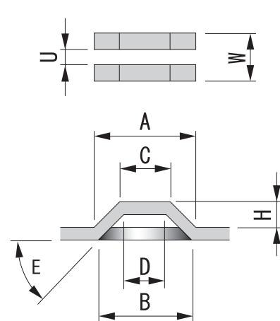
ダブルブリッジ（上向）
