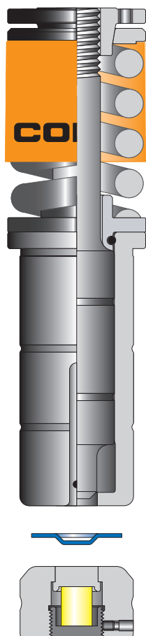
下向加工
