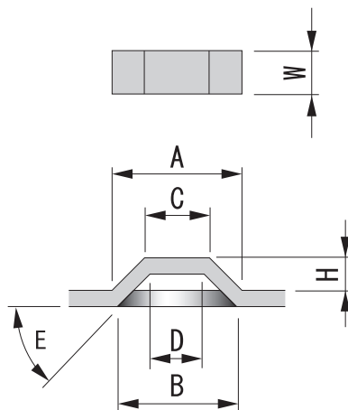
シングルブリッジ（上向）
