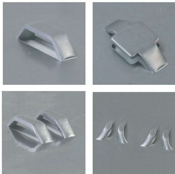
金型構造例 (NC 1-1/4)
