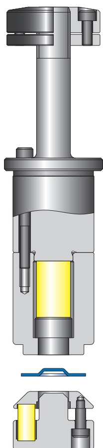
上向加工
