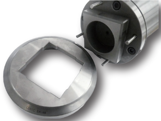
Est(4-1/2") 用芯出し治具セット例
