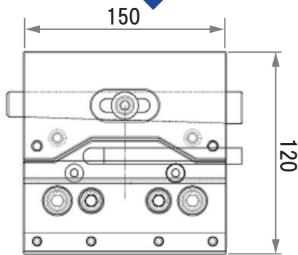
寸法図
