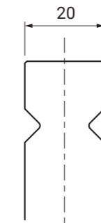
アイクランプ溝
